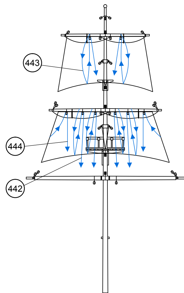
Aparejo de velas / Sail rig / Gréement Segel takelage / Sartieme da vela
